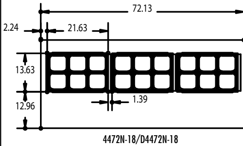
4472N-18/D4472N-18
